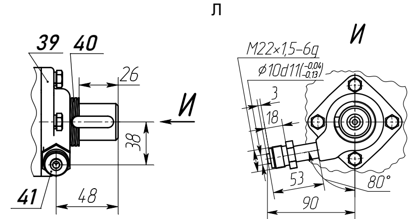
Рисунок А.4 - Вспомогательное уплотнение для одинарного торцового уплотнения (остальное см. рисунок А.1)
