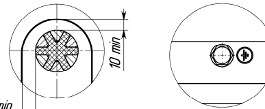
А-А (1:4) В Заземление базового двигателя
