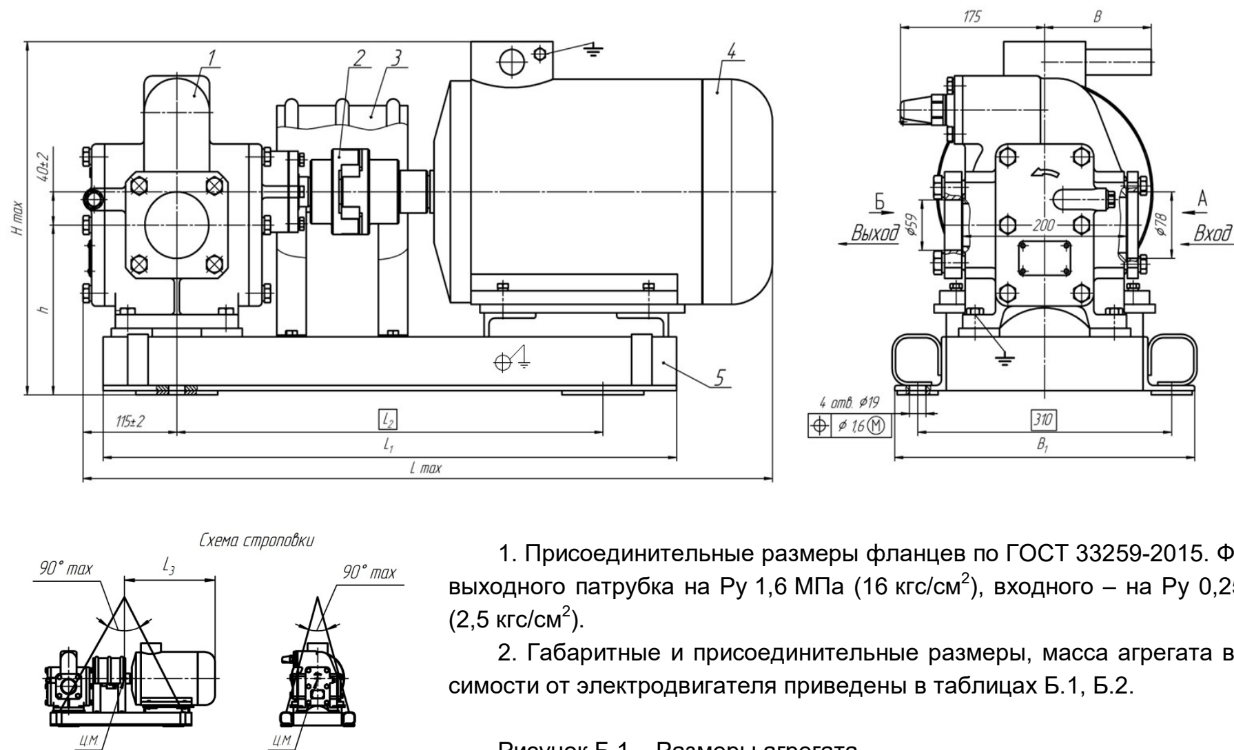
Рисунок Б.1 – Размеры агрегата
