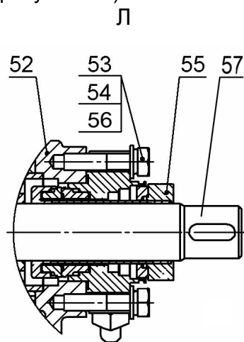
Рисунок А.5 - Двойное торцовое уплотнение (спина к спине) (остальное см. рисунок А.1)
