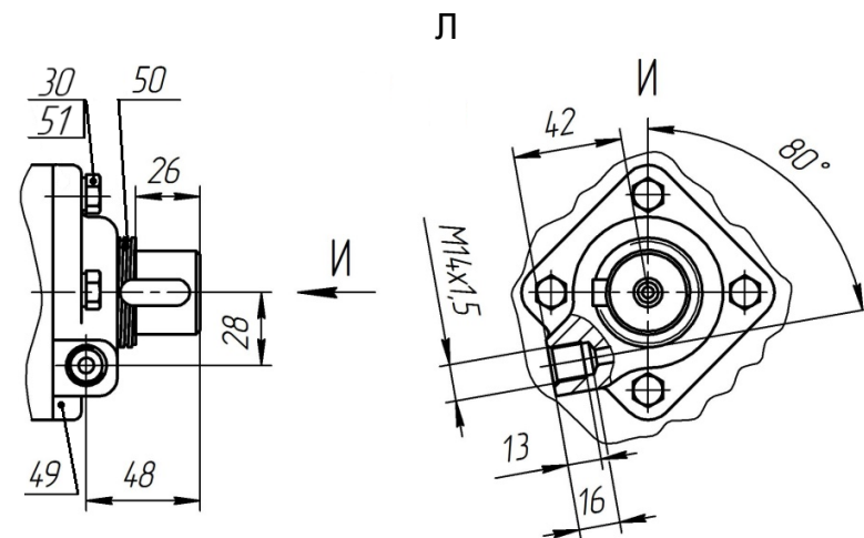
Рисунок А.4 - Дополнительное уплотнение для одинарного торцового уплотнения (остальное см. рисунок А.1)
