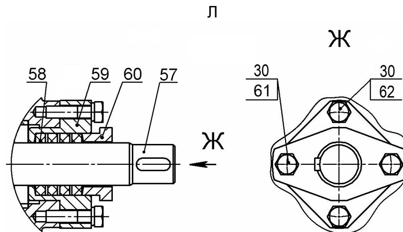
Рисунок А.4 - Дополнительное уплотнение для одинарного торцового уплотнения (остальное см. рисунок А.1)
